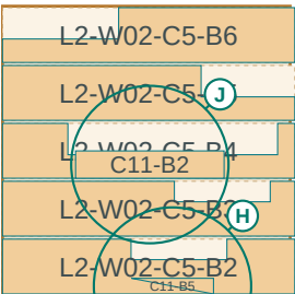
LAYER 6 - L2 courses 5, 11
