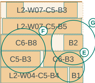
LAYER 7 - L2 courses 5-6
